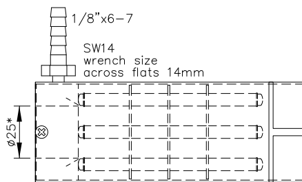
*: Lichter Durchmesser *: diameter inside
