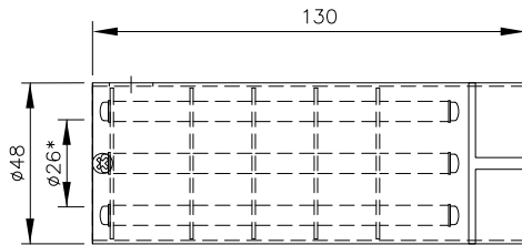
Tubusrohr mit Staubkäfing Tube with Dust Collector
