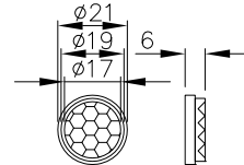
Typ / Type: R101 Best.-Nr. / Order no.: 6150 Befestigung / Mounting: Kleben / Glueing
