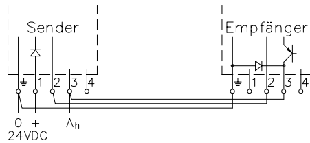
Anschlußplan
